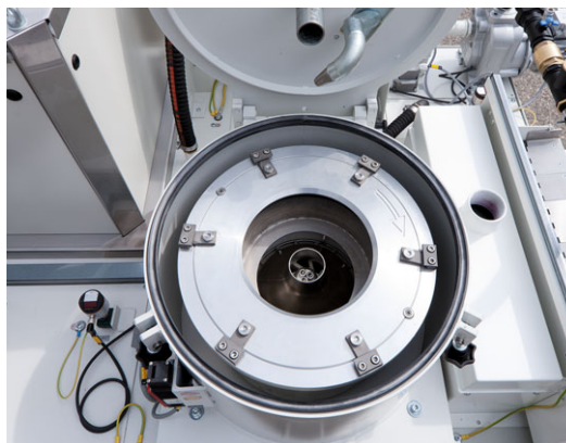
Duplafalú dobszűrő centrifuga TZ
